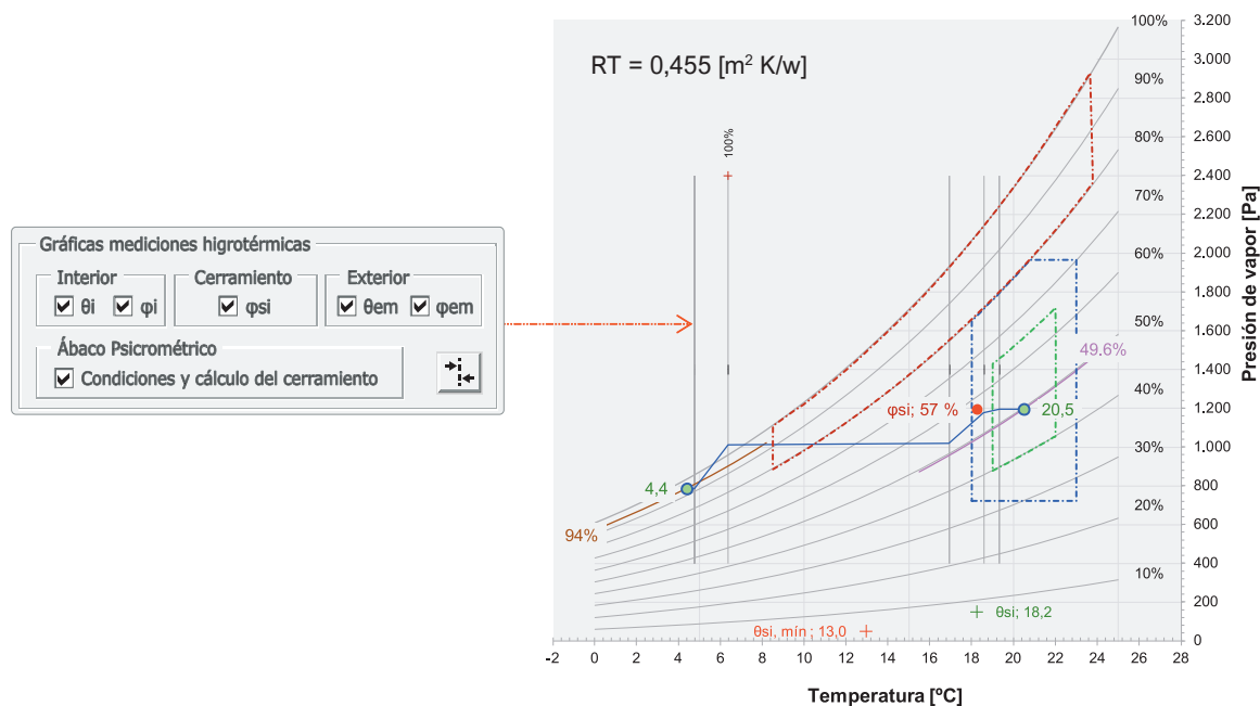
Imagen 68. Resultados del cerramiento en el Ábaco Psicrométrico.
