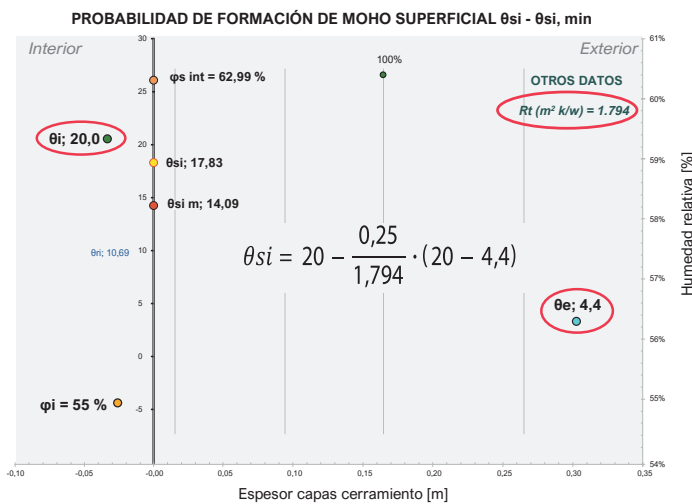
Imagen 29. Cálculo \theta_{si}
