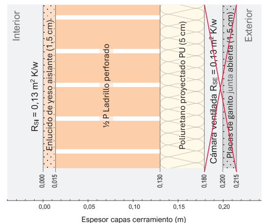
Imagen 13. Esquema del cálculo de la resistencia térmica de cerramiento con cámara de aire muy ventilada.
