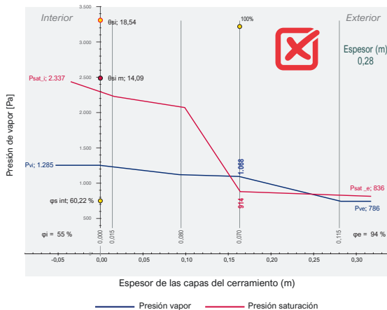
Imagen 36. Cruce de gráficas: riesgo de condensación intersticial.
