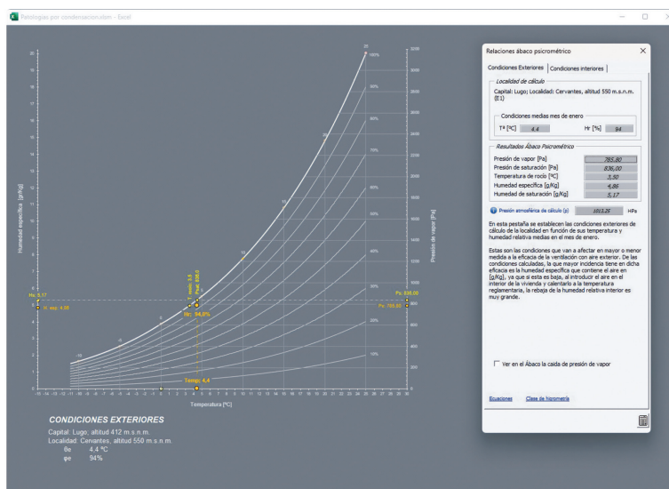
Imagen 140. Ábaco psicrométrico.
