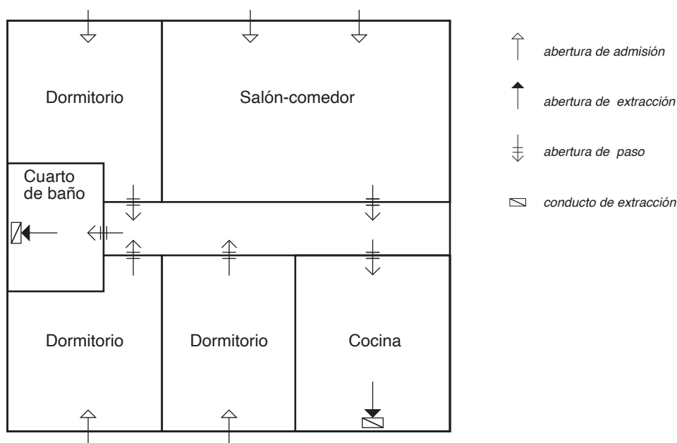
Imagen 106. Esquema de ventilación descrito en el DB HS3 Calidad del aire interior.
