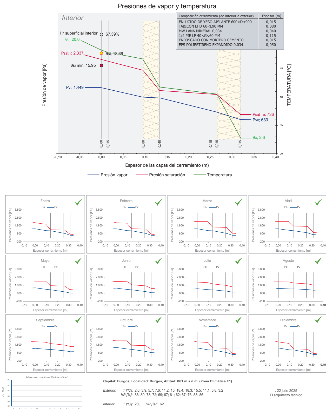
Imagen 46. Solución con un Sistema de Aislamiento Térmico por el Exterior (SATE).
