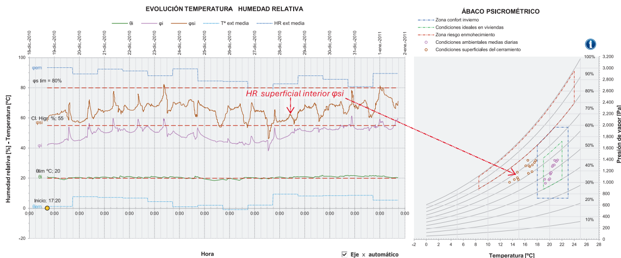
Imagen 67. Gráfica calculada de humedad relativa superficial interior \phi_{si}
