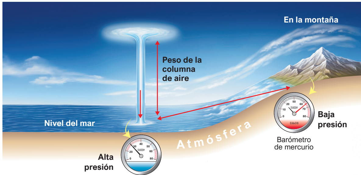
Imagen 1. Presión atmosférica.
