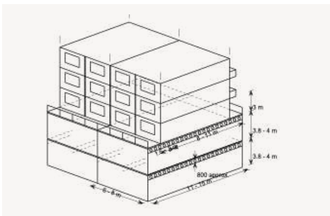
Fig 53. Módulos apoyados en vigas alveolares de gran longitud (SCI).
