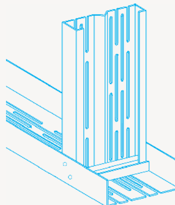
Fig 28. Muro portante utilizando una estructura de acero ligero con montantes ranurados (SCI).
