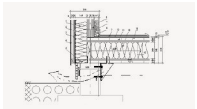
Fig 38. Detalle de unión de los módulos y la cimentación propuesto por en el proyecto de Biarritz Parme Francia de la empresa Egoín.
