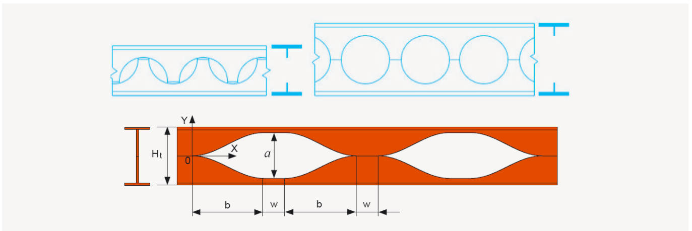
Fig 10. Ejemplo de perfiles aligerados. Fuente. Arcelor Mittal.
