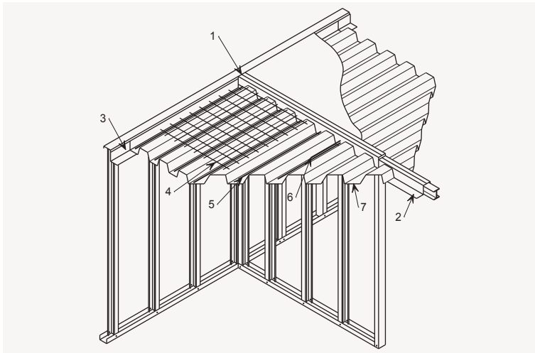
Fig 26. Forjado de acero y de hormigón adecuado para forjados divisorios en apartamentos de varias plantas (Acces Steel).
