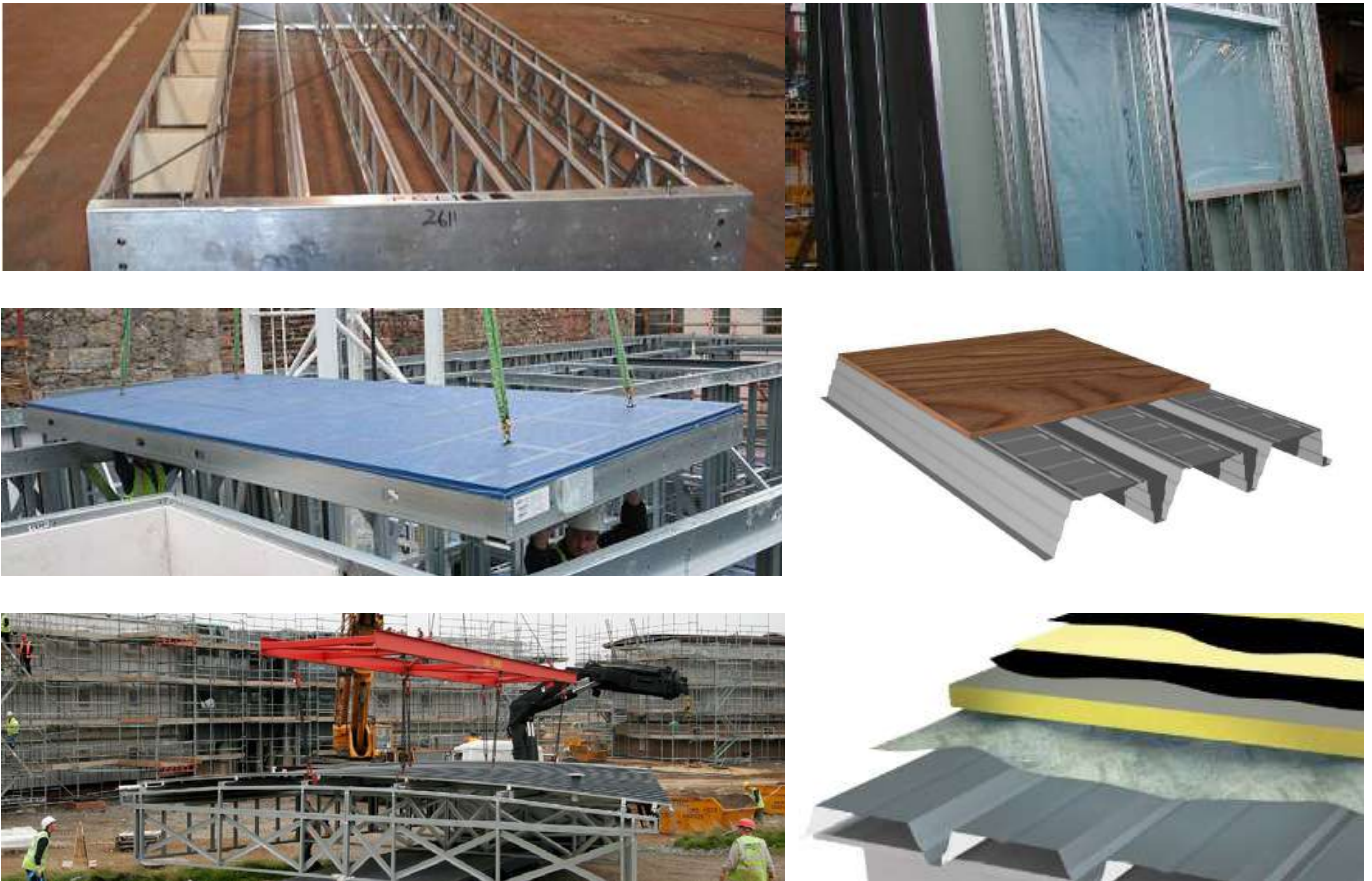
Fig 20. Ejemplos de construcción de paneles conformados en frío.
