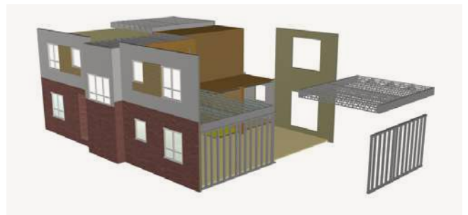
Fig 51. Combinación de módulos, forjados y paneles (Proyecto Europeo RFCS).
