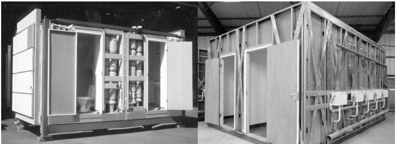
Fig 41. Ejemplos de construcción modular para servicios o baños en base a acero. (Fuente: SCI-P302 y P130).
