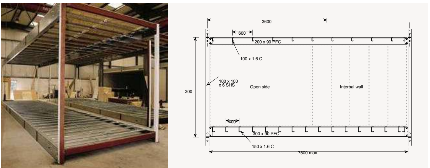
Fig 44. Estructura principal de módulos abiertos (Kingspan).
