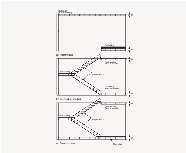
Fig 49. Representación gráfica de tres módulos de escaleras con falsos descansillos (SCI).
