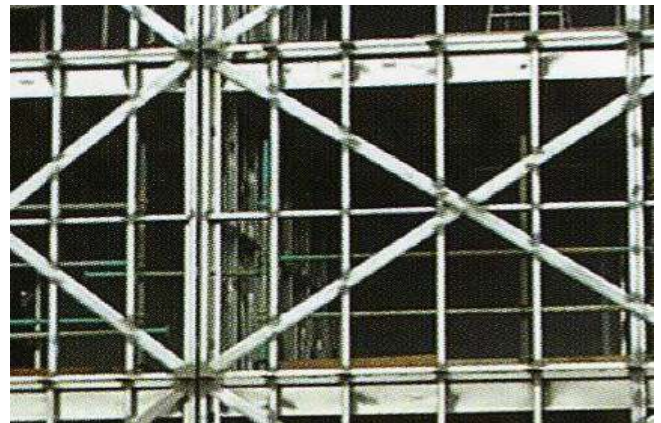
Fig 27. Muro estructural con arriostramiento en cruz de San Andrés (SCI).
