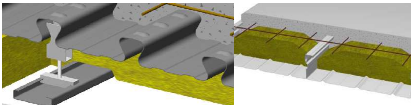
Fig 25. Sistemas de forjado Cofastra Decibel y Cofradal (Arval).
