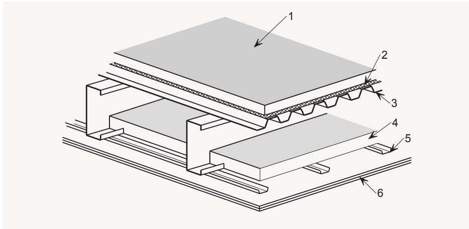
Fig 23. Forjado de acero ligero con perfiles en C y una chapa de acero perfilado en la parte superior (Acces Steel).
