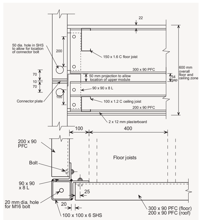
Fig 47. Unión de las vigas de borde y pilares tubulares en esquinas (SCI-P348).
