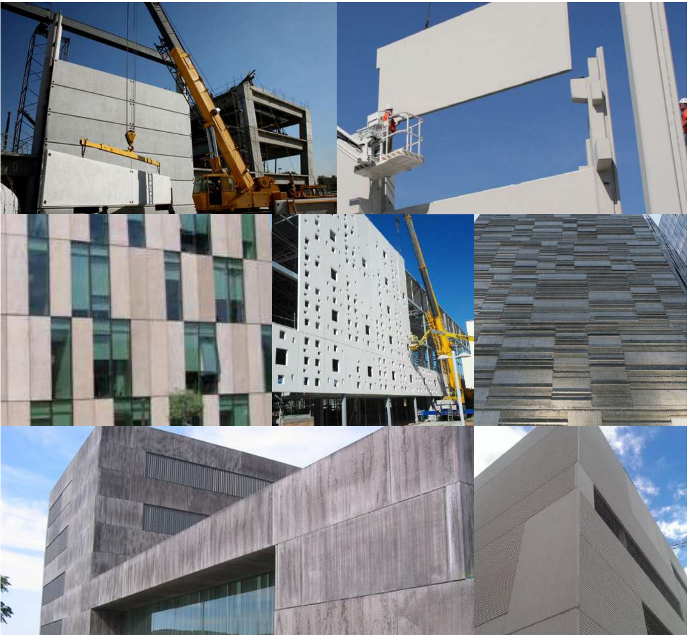
Fig 34. Paneles de hormigón prefabricado tanto en edificios industriales como en residenciales o terciarios.
