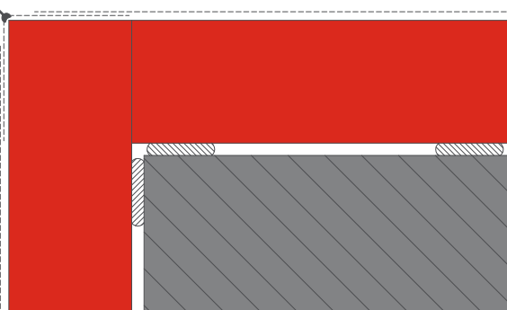
Detalle malla con esquinero flexible
