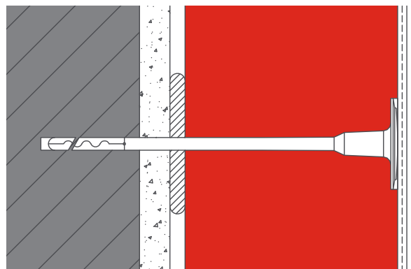
Exterior frío
