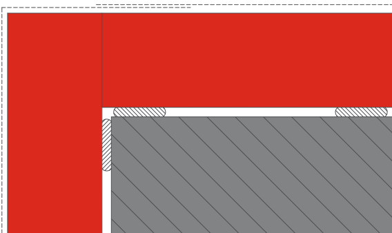
Detalle malla en refuerzo en esquina
