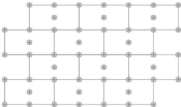
Detalle de anclaje con fijación
