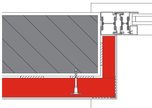
Detalle ventana
