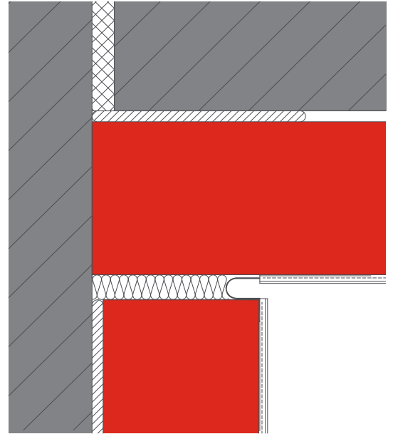
Detalle juntas de dilatación en esquina
