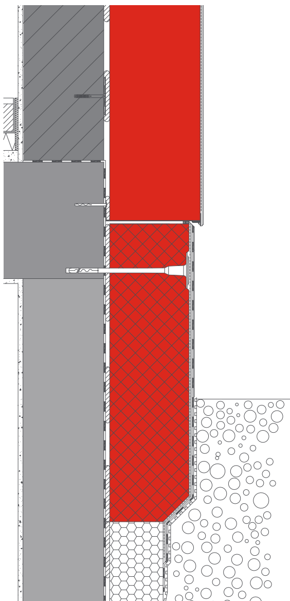
Detalle zona de salpicadura en zócalo con perímetro de aislamiento
