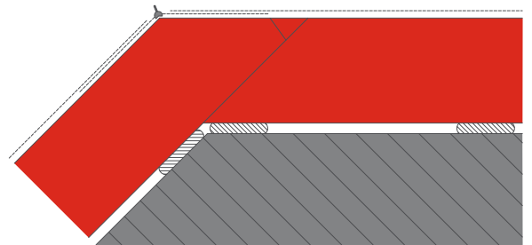
Detalle malla de armadura con esquinero
