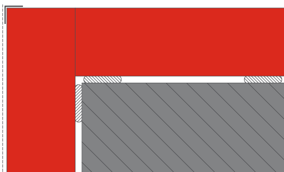
Detalle malla con esquinero
