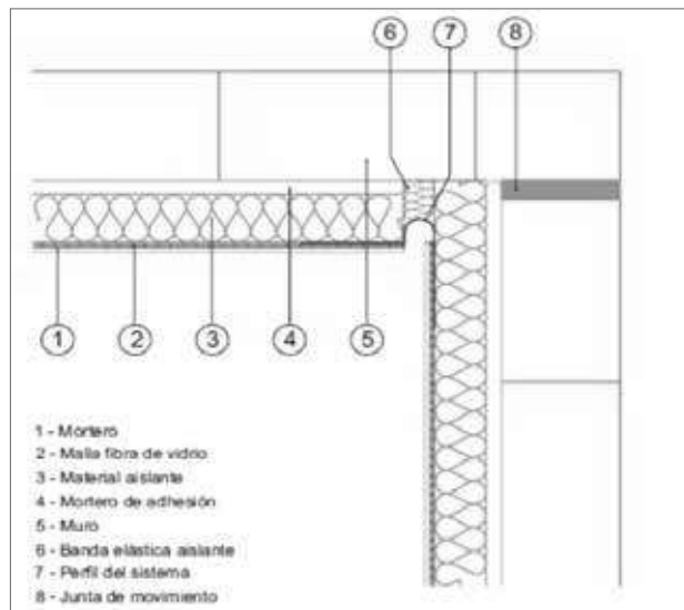
Detalle 7. Junta de dilatación en rincón.
