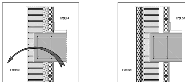
Puente térmico cuando el aislamiento está por el interior.
