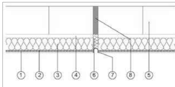
Detalle 6. Junta de dilatación.
