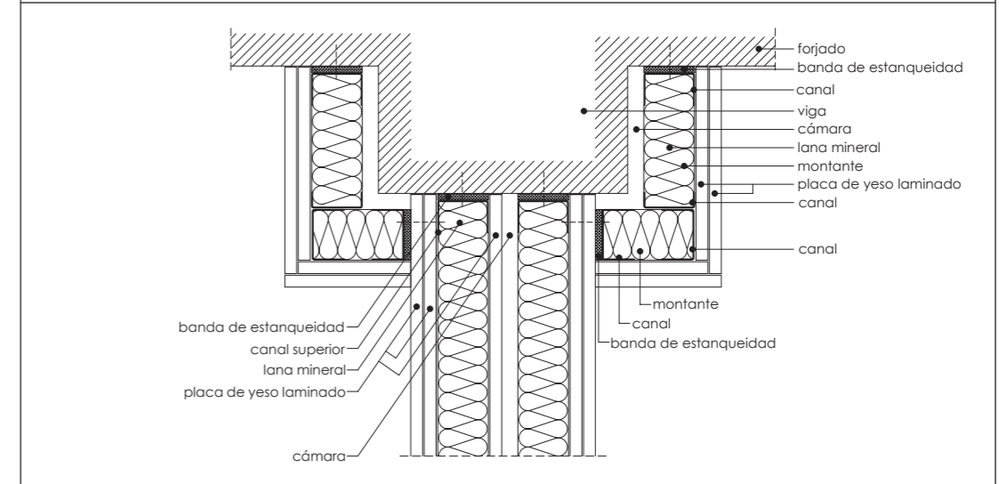
K.8.4. Vigas
