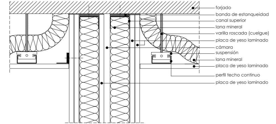
K.7.1. Solución PYL
