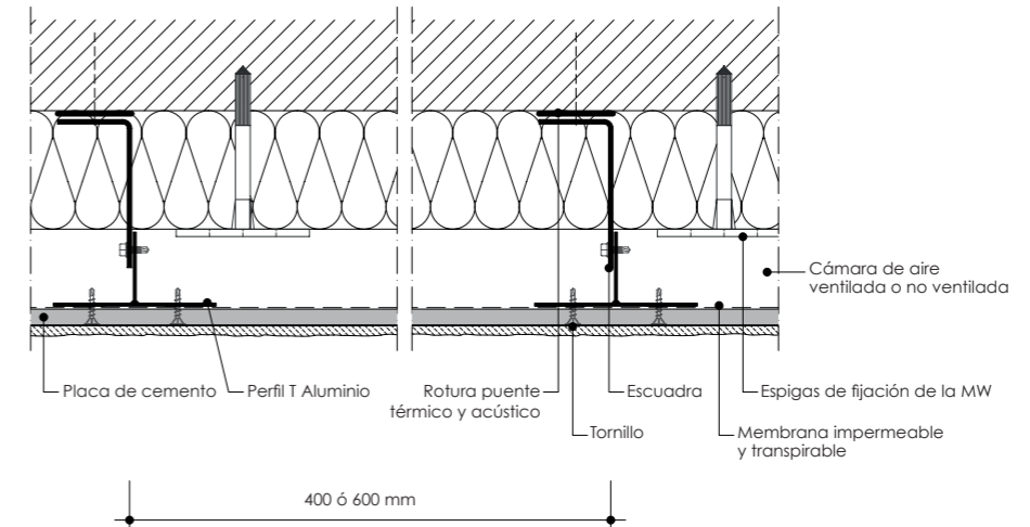
K.10.2. Sección horizontal fachada ventilada o no ventilada
