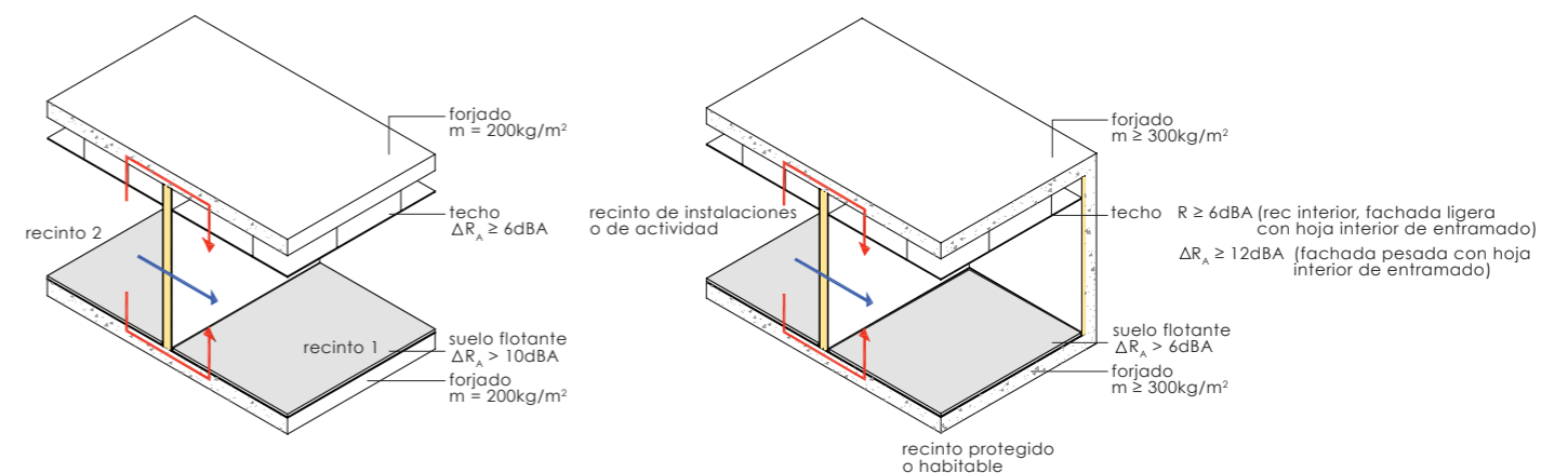
Figura 1. Condiciones de los techos y suelos flotantes para la utilización de los elementos de separación verticales de PYL entre un recinto protegido y un recinto de actividad o instalaciones. Guía del DB HR Protección frente al ruido. Versión V.02
