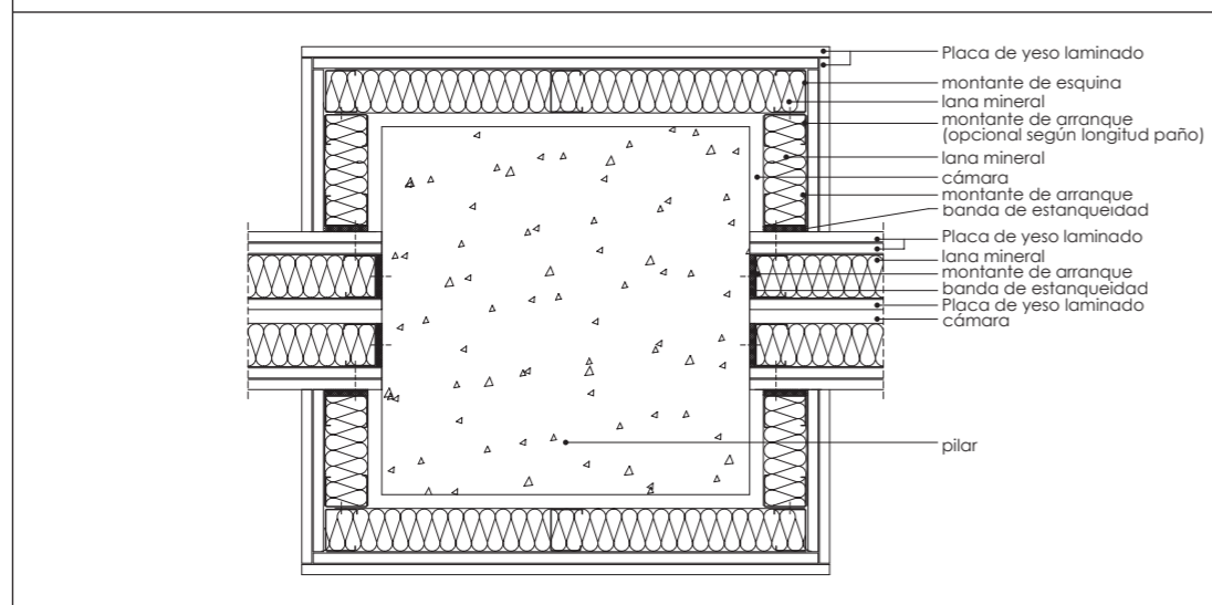
K.8.3. Pilares
