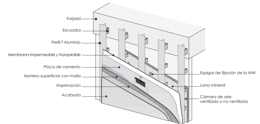
K.10.1. Esquema fachada ligera
