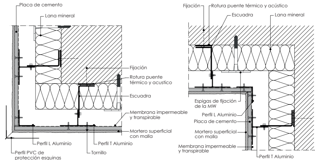
K.10.3. Solución esquina y rincón
