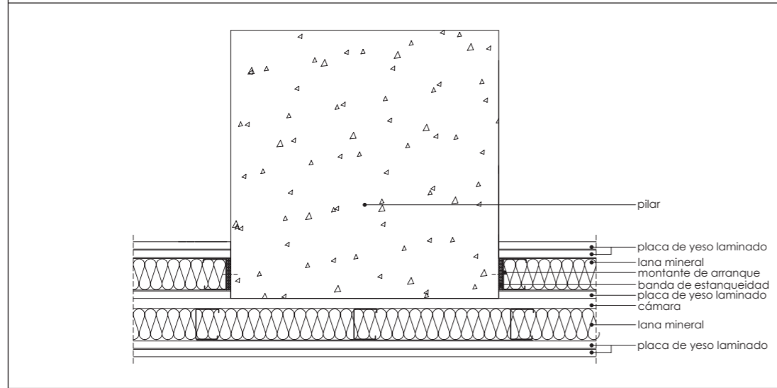
K.8.1. Pilares
