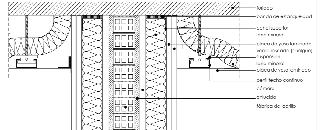
K.7.2. Solución mixta
