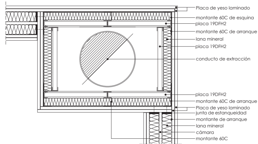
K.9.2. Solución para patinillos de extracción de humos de garaje
