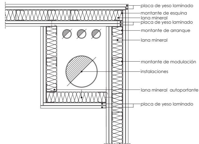
K.9.1. Solución para patinillos de instalaciones
