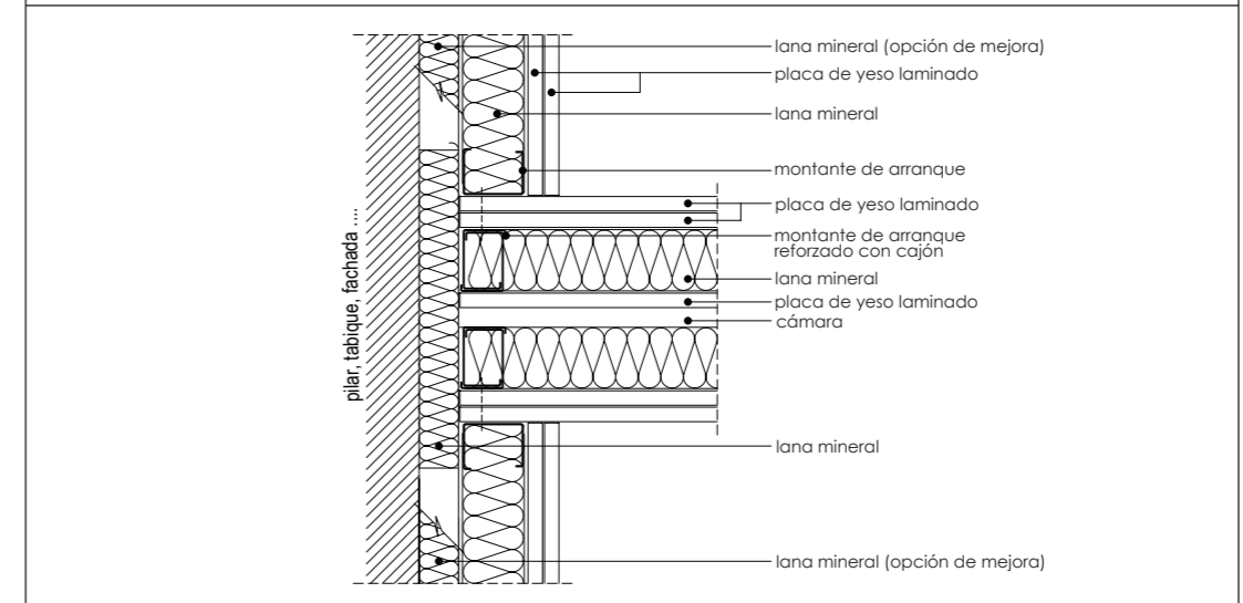
K.8.5. Variante de solución de arranque de pilar o muro - Solución autoportante
