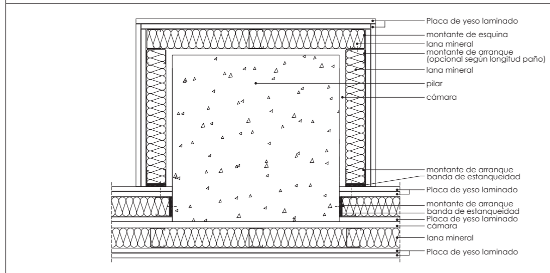
K.8.2. Pilares
