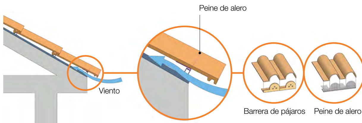
Figura 54. Funcionamiento de entrada de aire por alero con barrera de pájaros o peine de alero
