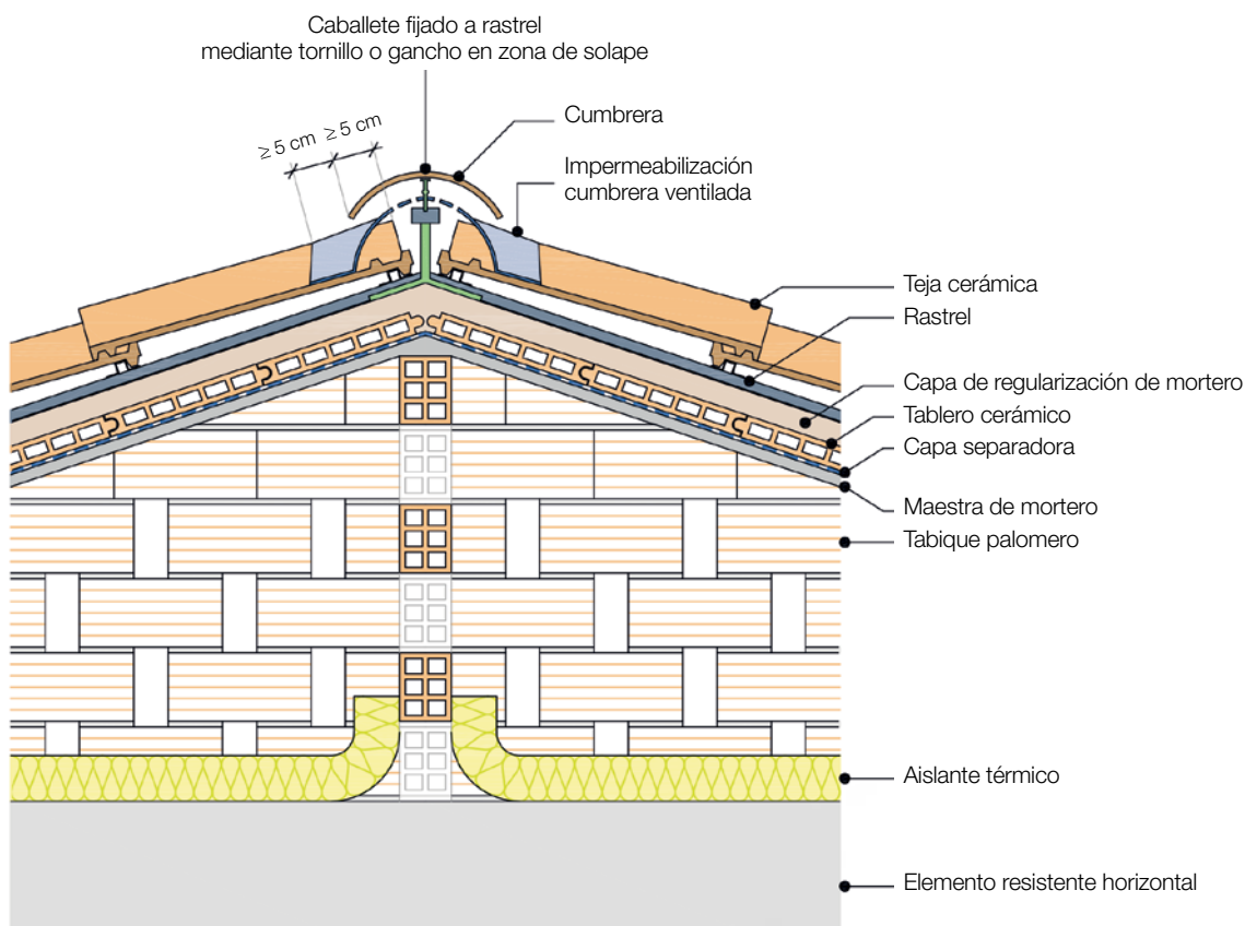
Figura 73. Cumbrera de una cubierta QB12
