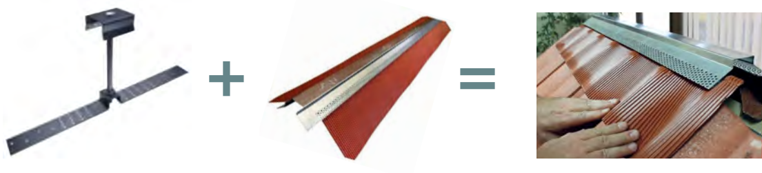
Figura 75. Soporte de caballete del tipo perfil metálico ranurado con forma de rastrel y sus componentes
