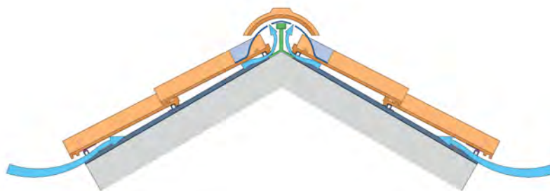
Figura 3. Remate de cumbre
