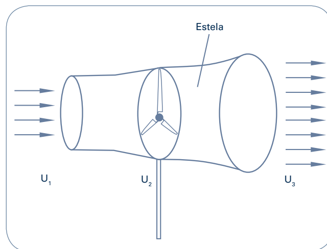
FIGURA 1 Tubo de corriente de la aeroturbina en la teoría unidimensional de Betz.
