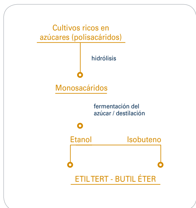
FIGURA 13 Proceso de producción de ETBE.
