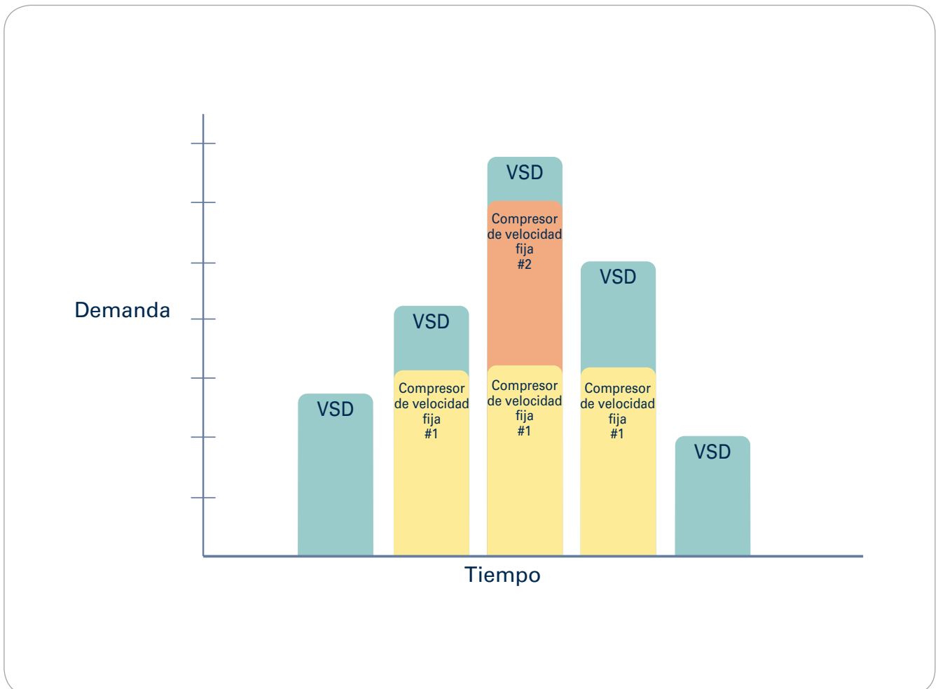
FIGURA 4 Fraccionamiento de la potencia de los compresores.
