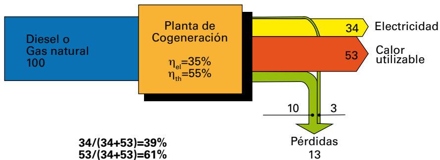
Esquema de abastecimiento energético con cogeneración.
