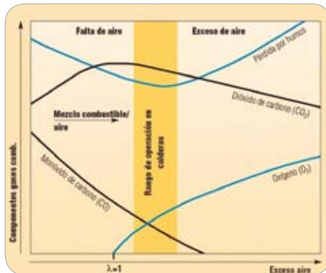
FIGURA 7 Parámetros óptimos del aire de combustión (Cortesía Testo).
