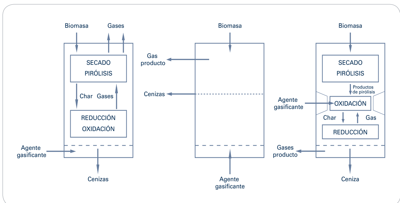
FIGURA 3 Esquemas de funcionamiento de gasificadores: de izquierda a derecha: gasificador updraft , gasificador de lecho fluidizado y gasificador downdraft .
