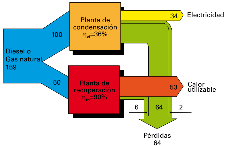
Esquema de abastecimiento energético convencional.
