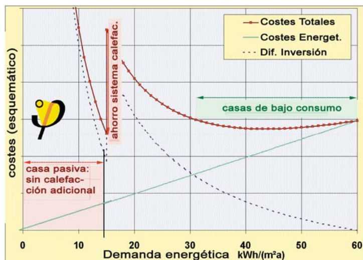
Gráfico 1. Costes acumulados a 20 años. Fuente: Passive House Institute.
