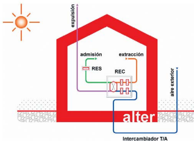
Figura 4. VMC con recuperación y resistencia eléctrica. Fuente: Alter Technica.
