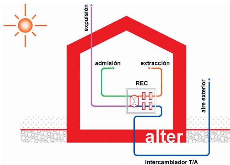
Figura 3. VMC con recuperación e intercambiador tierra/aire. Fuente: Alter Technica.
