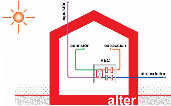
Figura 2. Esquema básico VMC con recuperación. Fuente: Alter Technica.
