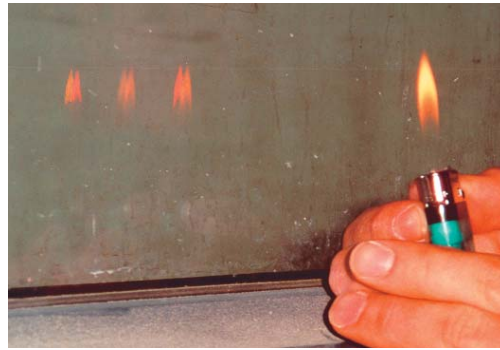
Fotografía 3. Imagen de comprobaciones en obra de la posición de las láminas en los vidrios Fuente «Passivhäuser im Sonnenfeld» Autores Joachim Zeller y Claus Kahlert.
