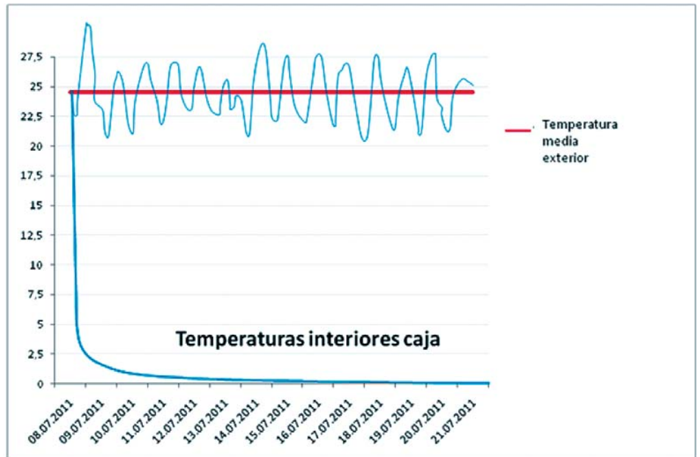
Gráfico 3. Temperaturas interiores de la caja. Fuente: Micheel Wassouf, TBZ.
