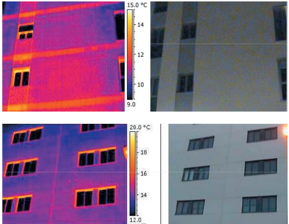
Fotografía 1. Frentes de forjado sin aislamiento y marcos de ventana sin rotura de puente térmico detectados en una inspección con termografía en el Ecobarrio de Valdespartera (Zaragoza).
