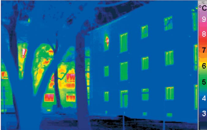
Fotografía 3. Termografía de viviendas. Fuente: Google.
