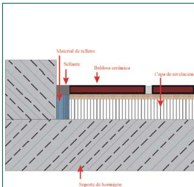
Junta perimetral en el encuentro del pavimento con cerramientos y particiones
