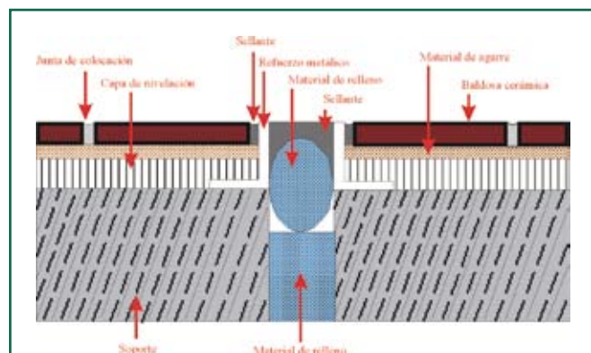
Junta estructural en un pavimento cerámico de tránsito no exclusivamente peatonal, con protección de los bordes de la baldosa
